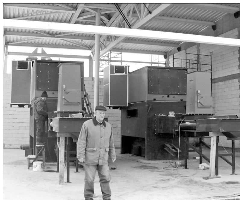
Kotłownia na biomasę w Jezierzycach
